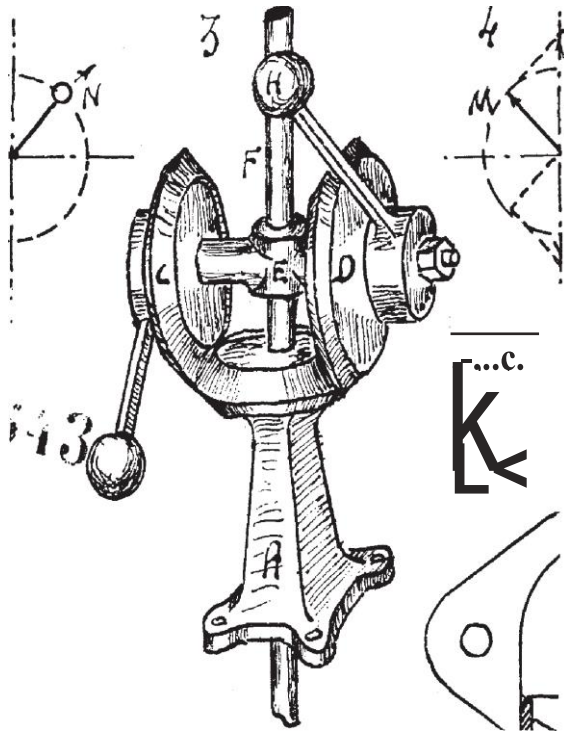
Motore a forza propulsiva centrifuga. G, H = Masse sferiche. C, D = Satelliti. A = Sostegno del planetario B fisso. F = Albero motore.
